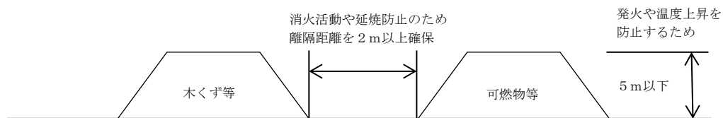
災害廃棄物の積み上げ高さ及び配置
