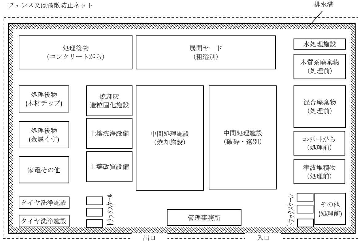
図3-9 二次仮置場レイアウト例
