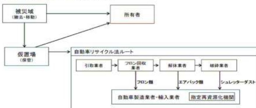
図2-3-13-3 被災自動車の処理フロー
