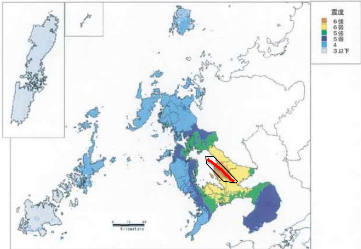
図2-2-1-10 地表における推計震度分布（震源：大村諫早北西付近断層帯）
