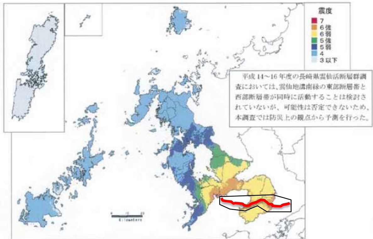
図2-2-1-9 地表における推計震度分布 (震源：雲仙地溝南縁東部断層帯と西部断層帯の連動)
