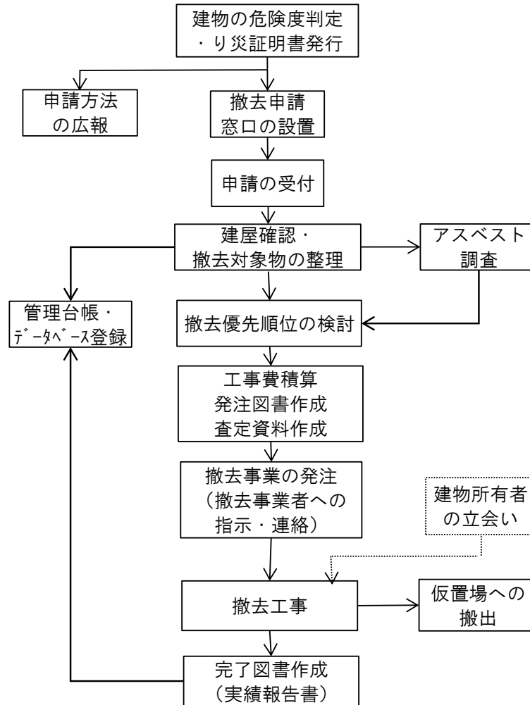
図 3-9 家屋・建屋の撤去手順（例）
